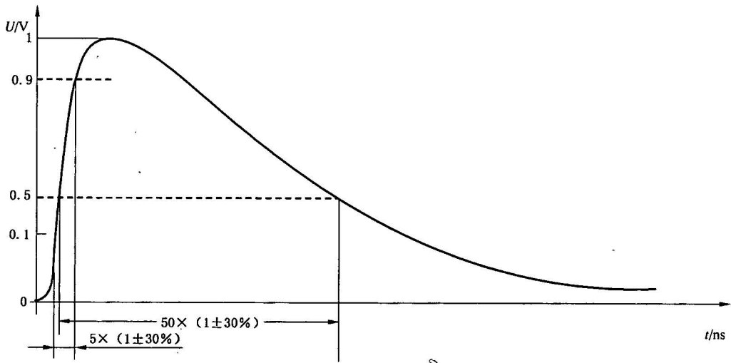
图 3 50Ω 负载时单脉冲波形
