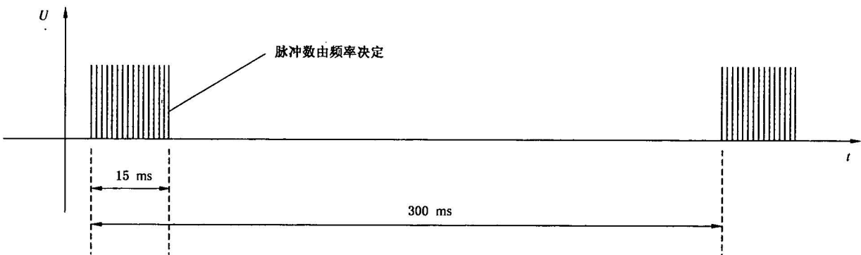
图 4 一组脉冲波形图
