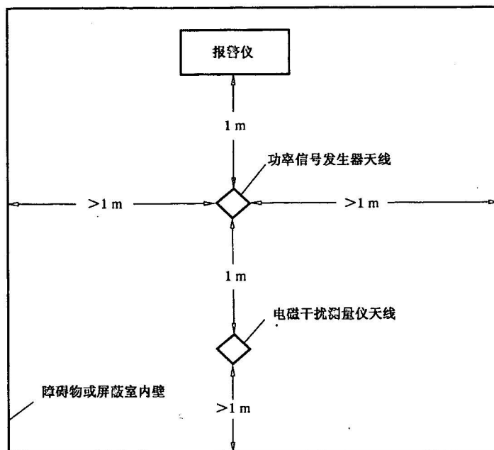
图2 天线位置图
